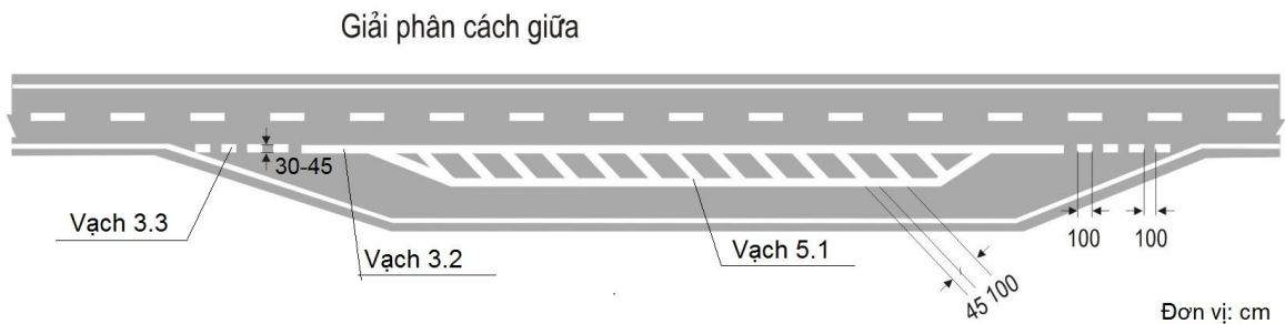
Hình G.19 - Bố trí vạch ở điểm dừng xe kiểu bến cảng, trường hợp sử dụng vạch 5.1 e. Bố trí vạch sơn trong khu vực bề rộng phần xe chạy bị thay đổi
