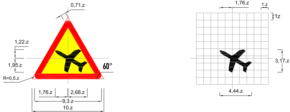
Biển số W.229: Dài máy bay lên xuống
