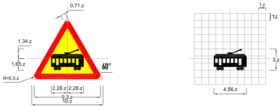
Biển số W.211b: Giao nhau với đường tàu điện
