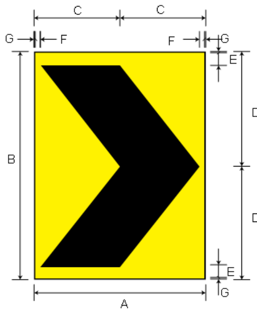
Hình 34 – Tiêu phản quang dạng mũi tên
