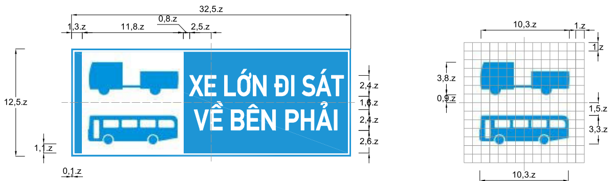
Biển số I.445e: Biển báo mô tả tình trạng đường
