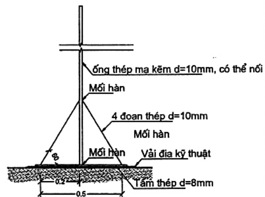
Bản vẽ chi tiết tấm sụt
